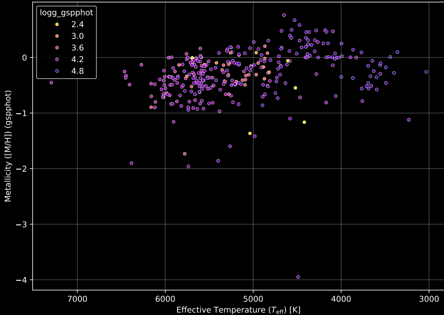
APOGEE DR17 Field: [066-79] Stellar Population Parameters (n= 313)
